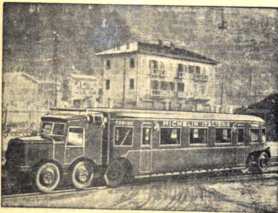
Schienenautobus,
